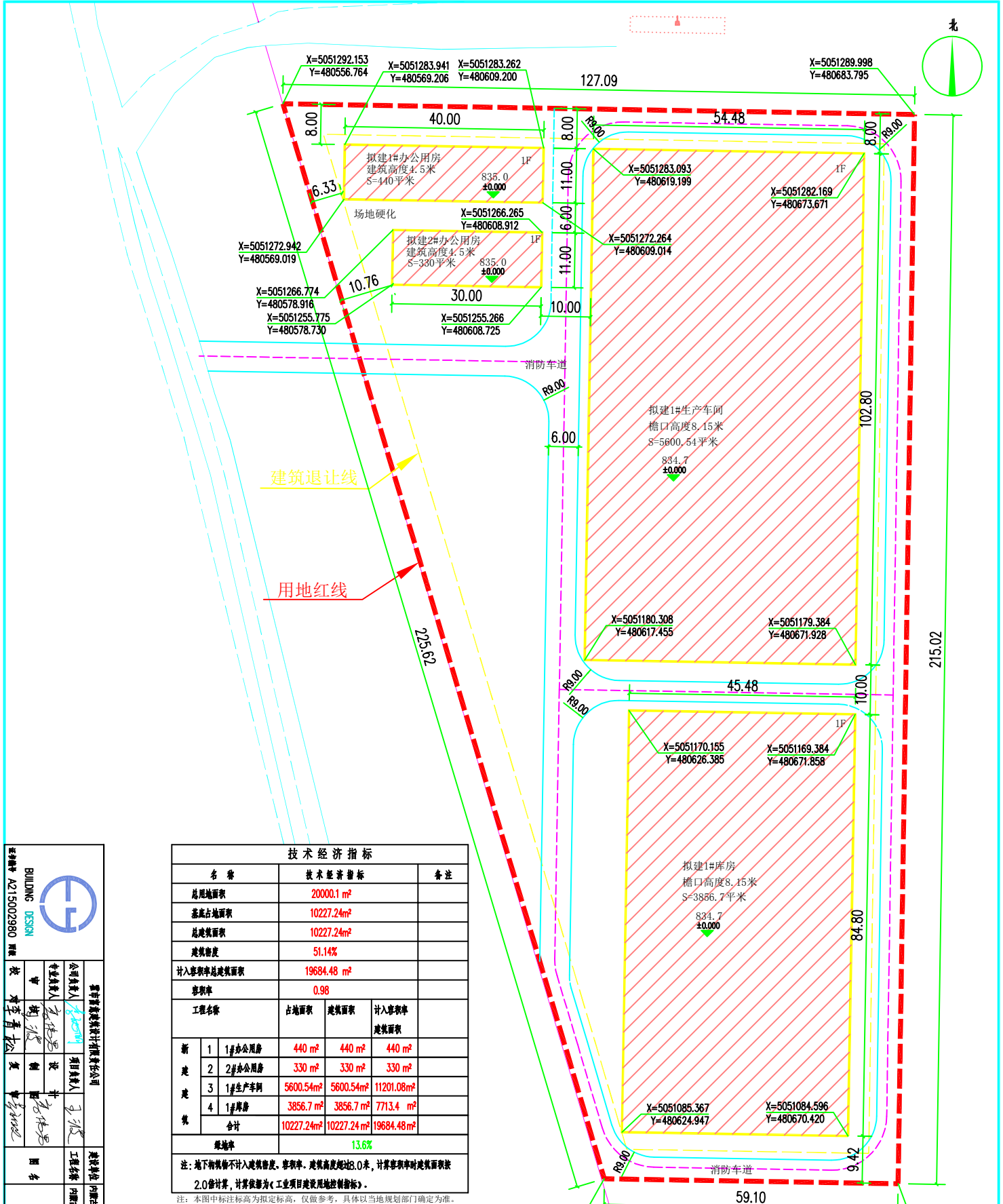
总平面图 1:500
